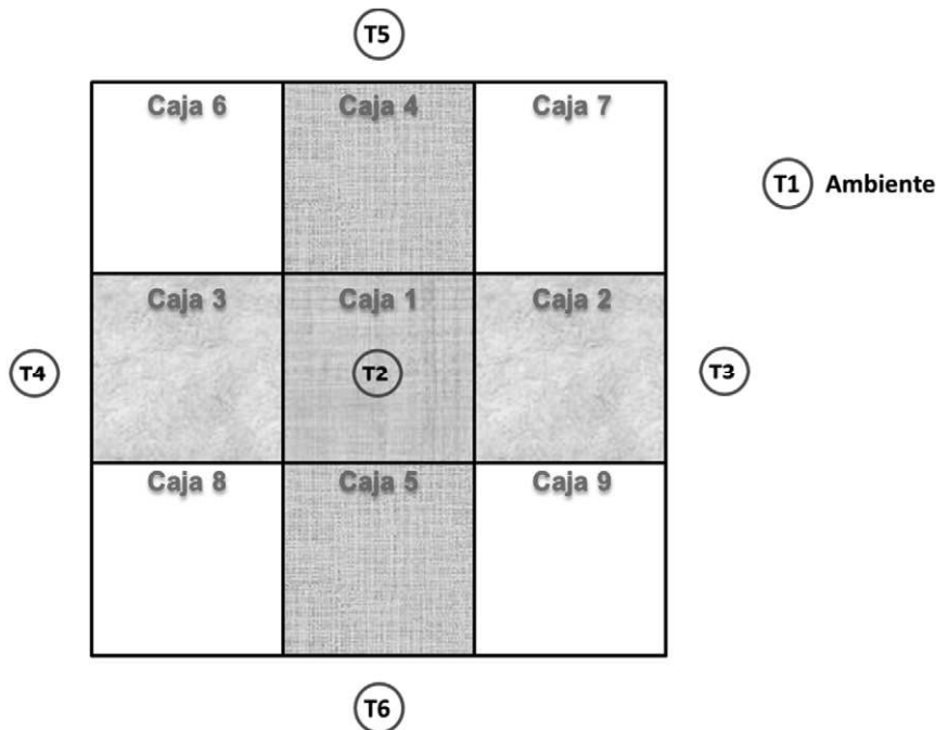
Figura 2. Esquema de colocación de termopares
